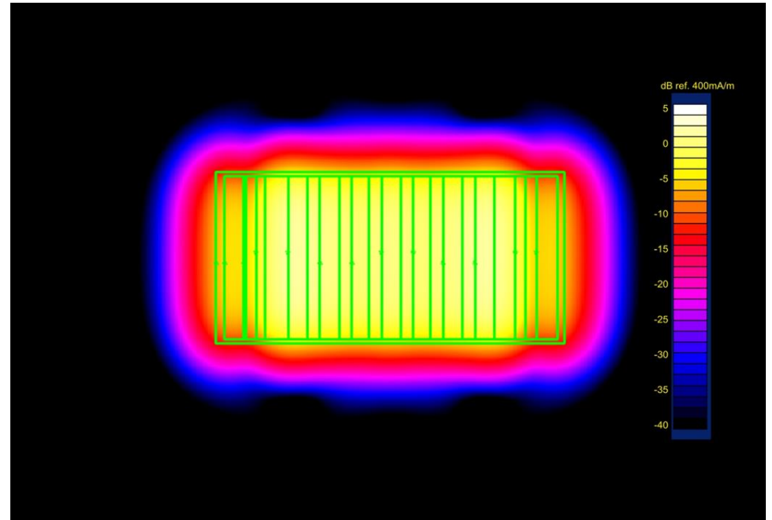
Vista en planta del campo magnético de audio de un bucle instalado en un auditorio.
